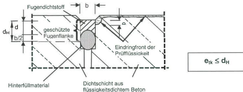
Bild 1: Umläufigkeitsverhalten im Bereich des eingebauten Fugenabdichtungssystems 1)
